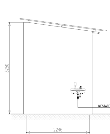
TAMPAK SAMPING Skala 1 : 30
