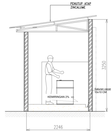
POTONGAN B Skala 1 : 30
